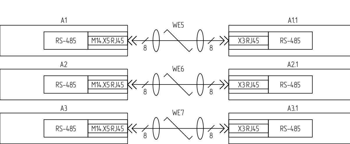
Цепи портов связи терминала
