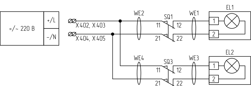
Цепи освещения шкафа
